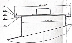
Узел IV М 10
